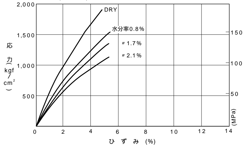
図-37 応力～歪曲線 (1300G)
