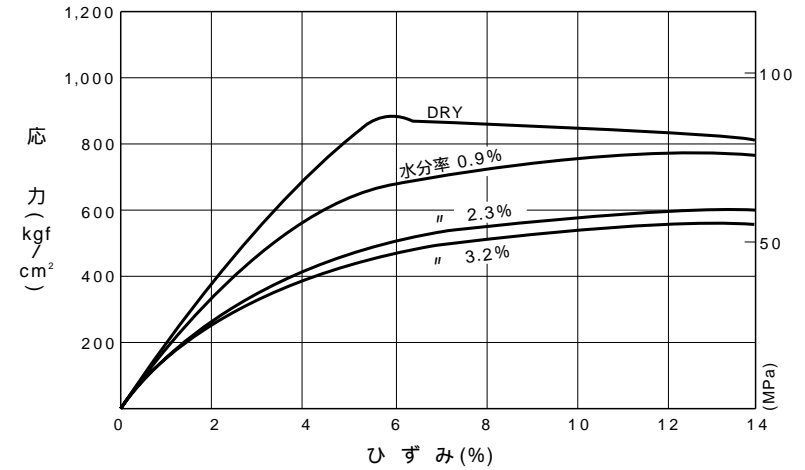
図-38 応力～歪曲線 (FR370)
