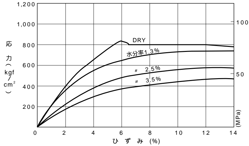
図-36 応力～歪曲線 (1300S)
